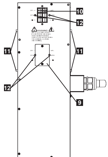
Задняя панель (применяется для всех 3 моделей)
